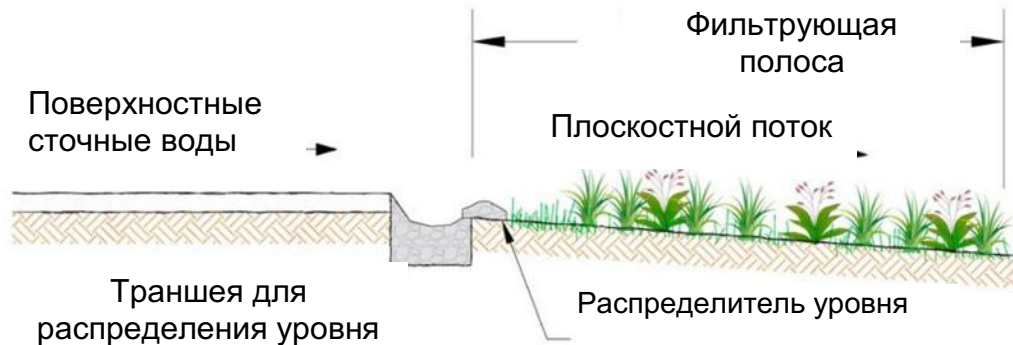
Рисунок 6 – Схема устройства фильтрующей полосы
