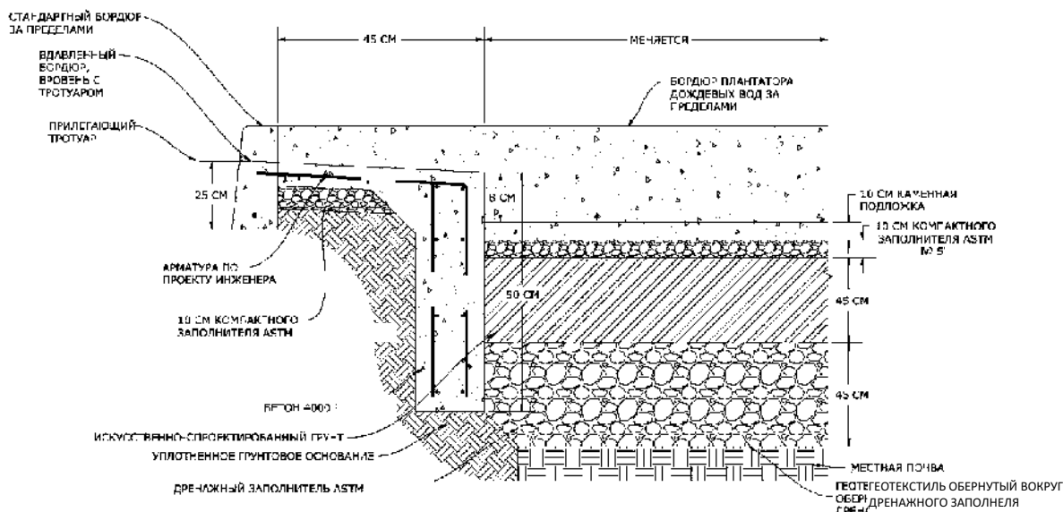
Рисунок 34 – Типовой профиль плантатора при обрезке бордюра
