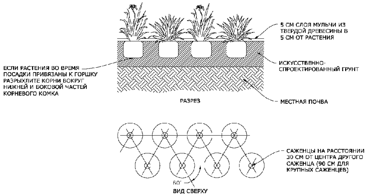
Рисунок 4 – Типовая схема рассадки растений в бассейне удержания типа «мокрый пруд»
