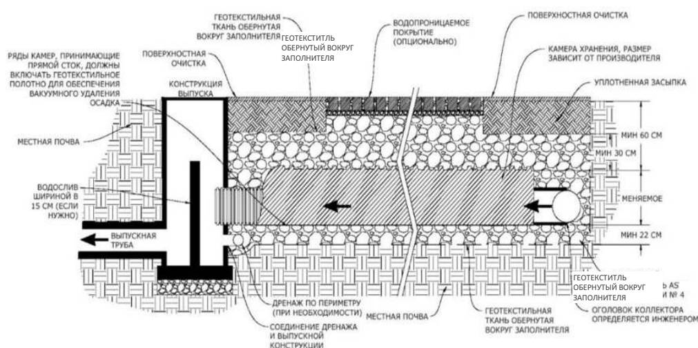
Рисунок 20 – Типовой профиль подземных накопителей
